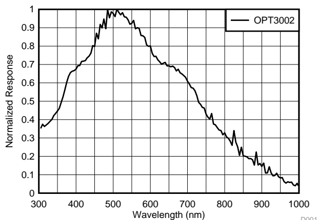
频谱响应
