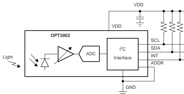
方框图
