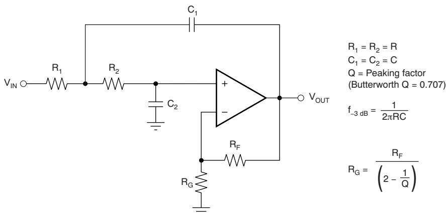
Figure 40. 两极低通 Sallen-Key 滤波器
