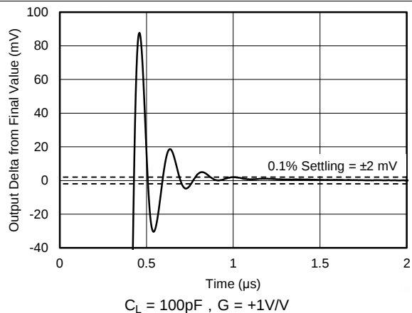
Figure 31. 正极性大信号趋稳时间
