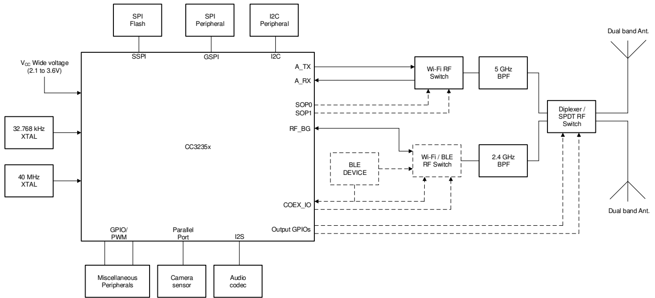
图 4-1. 功能方框图
