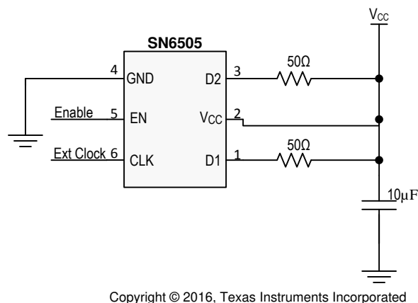
图 36. Test Circuit for F_{SW} , V_{(slew)} , t_{BBM}
