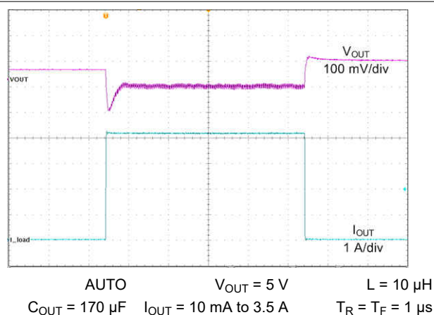
图 9-14. Load Transients
