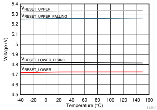
图 7-7. RESET Threshold Fixed 5-V Output
