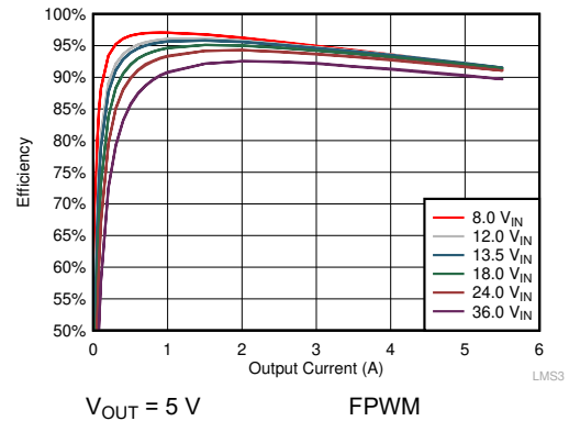
图 9-6. Efficiency
