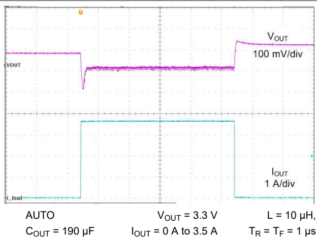
图 9-27. Load Transient
