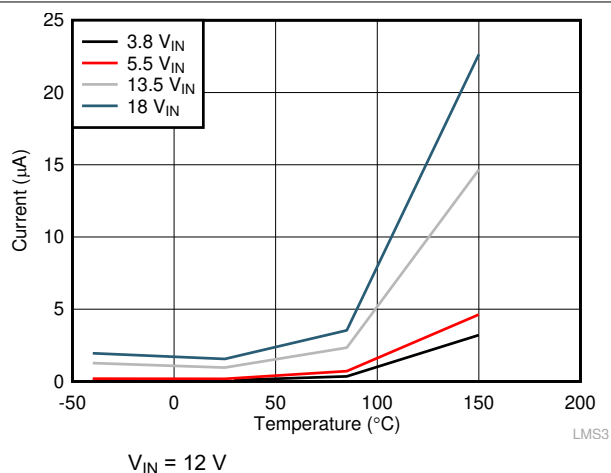
图 7-6. Shutdown Current
