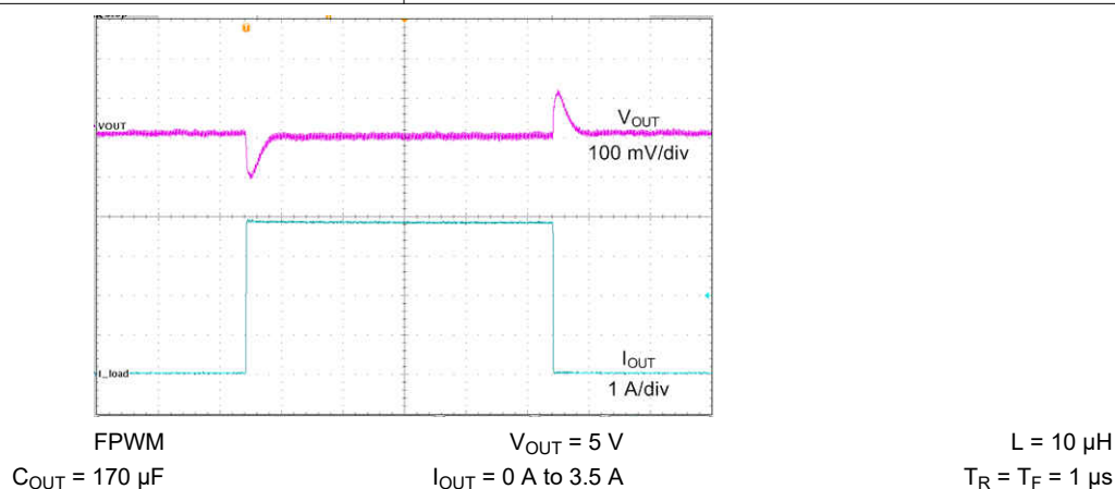
图 9-15. Load Transient
