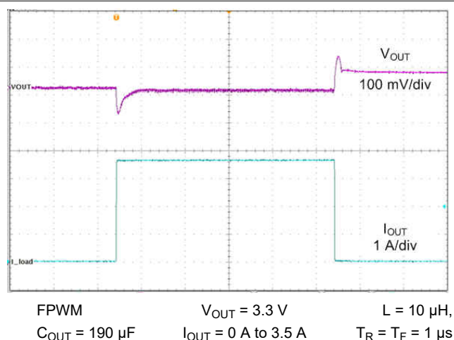
图 9-28. Load Transient
