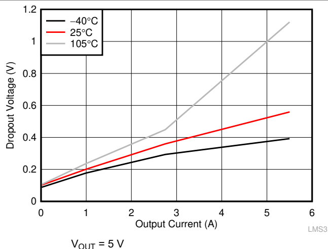
图 9-11. Dropout for \geq 330\text{ kHz}
