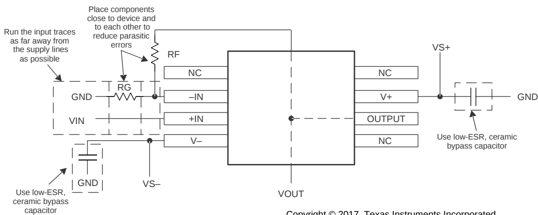
图 37. 同相配置的运算放大器电路板布局
