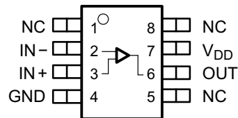
TLV2371-Q1 D 封装 8 引脚 SOIC 俯视图
