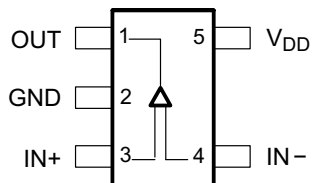
TLV2371-Q1 DBV 封装 5 引脚 SOT-23 俯视图
