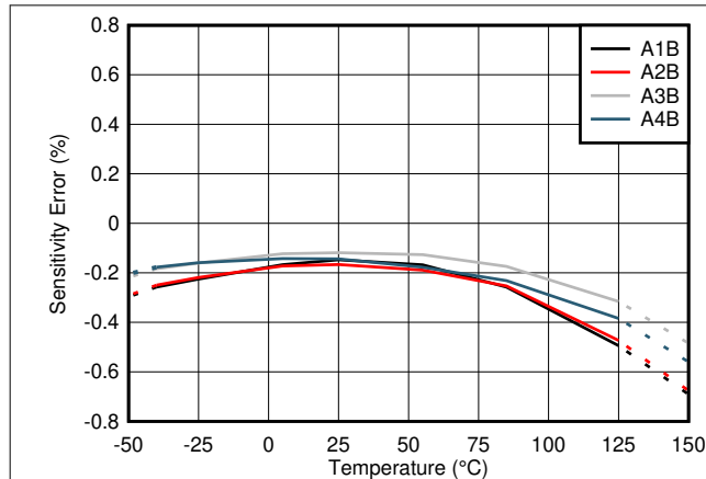
图 7-1. TMCS1101AxB-Q1 Sensitivity Error vs Temperature
