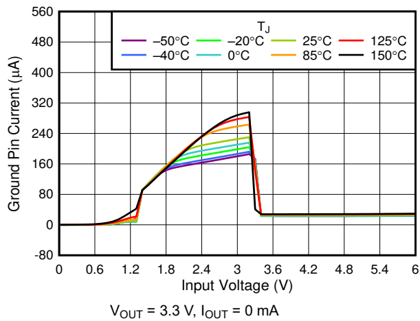
图 6-15. I_Q vs V_{IN}
