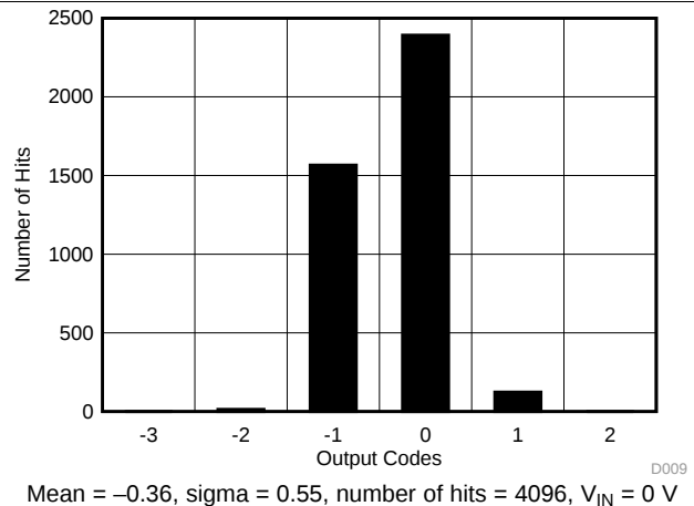
图 13. DC Histogram of Codes ( \pm 10\text{ V} )
