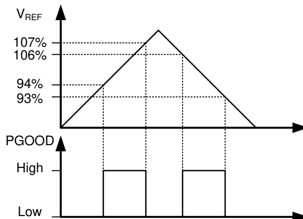
图 8-9. Power-Good Flag
