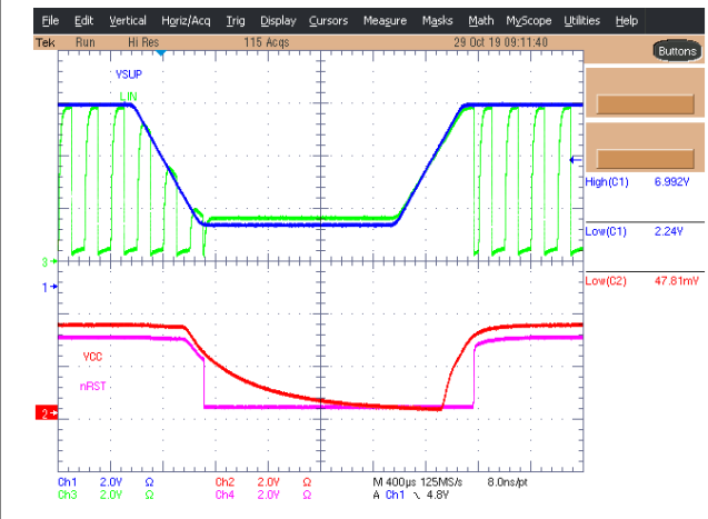
图 10-17. TLIN10283-Q1 Brownout
