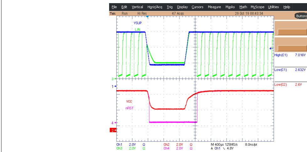
图 10-18. TLIN10285-Q1 Brownout
