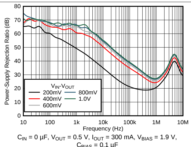
图 30. PSRR vs Frequency and V_{DO}
