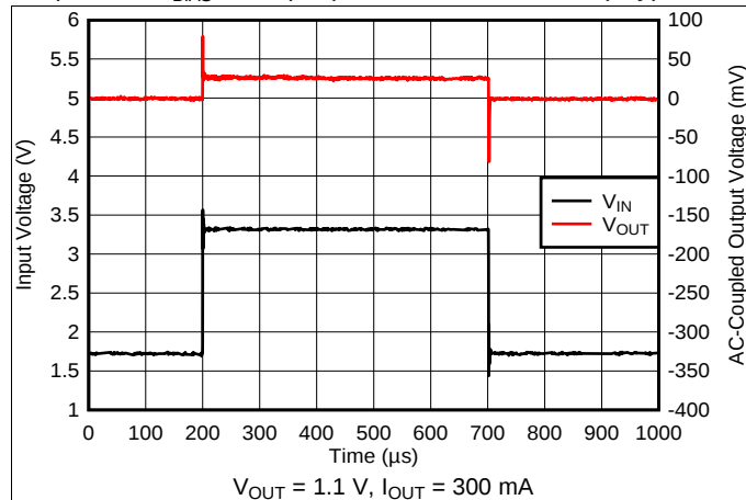
图 13. V_{IN} Transient
