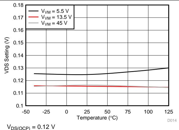
图 16. OCP Threshold Voltage
