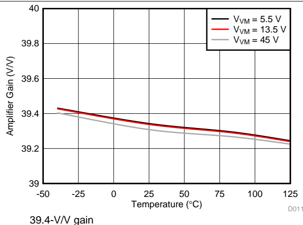
图 13. Amplifier Gain
