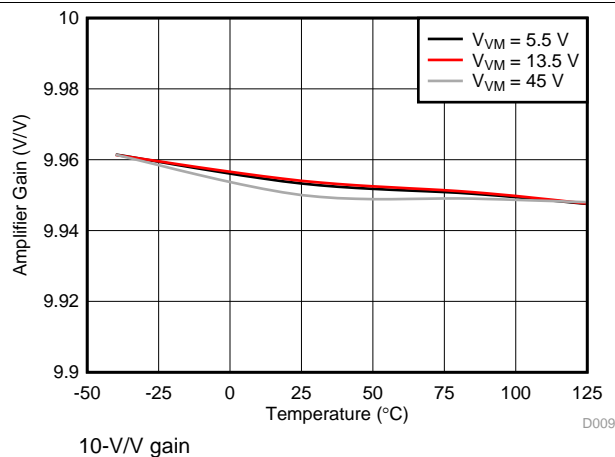
图 11. Amplifier Gain
