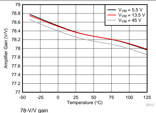
图 14. Amplifier Gain
