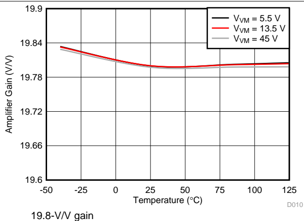
图 12. Amplifier Gain
