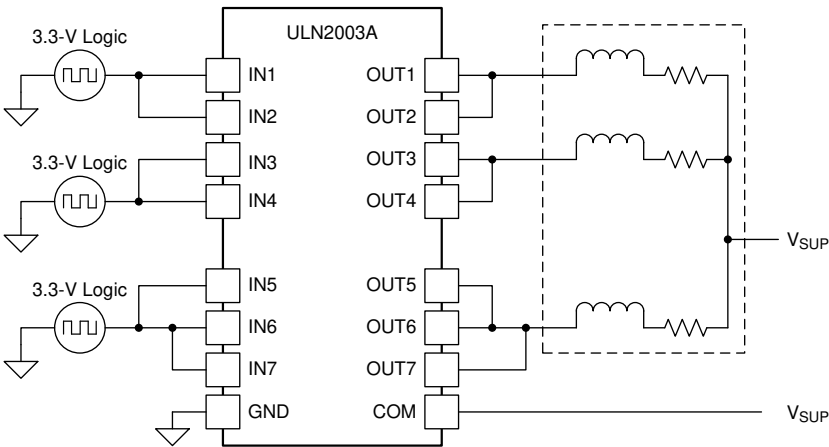
图 22. ULN2003A 器件用作感性负载驱动器
