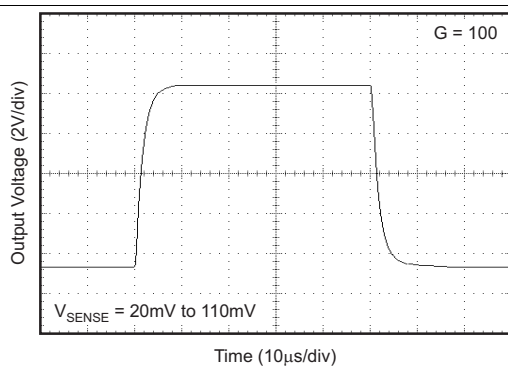
图 16. Step Response
