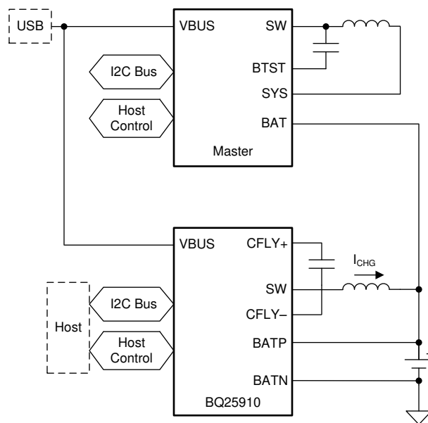
简化原理图
