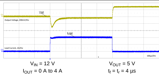
图 15. Load Transient
