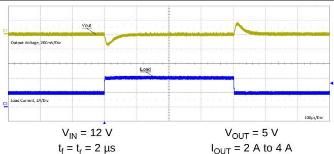
图 16. Load Transient
