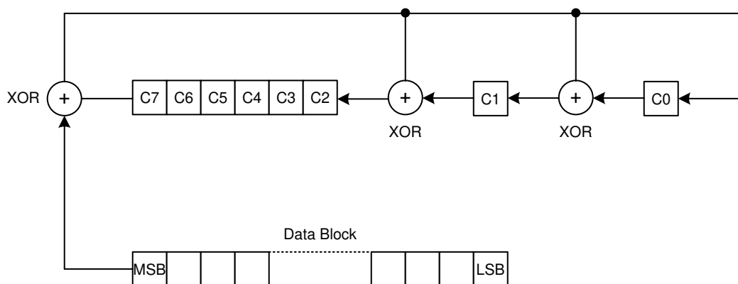
图 8-19. CRC Module
