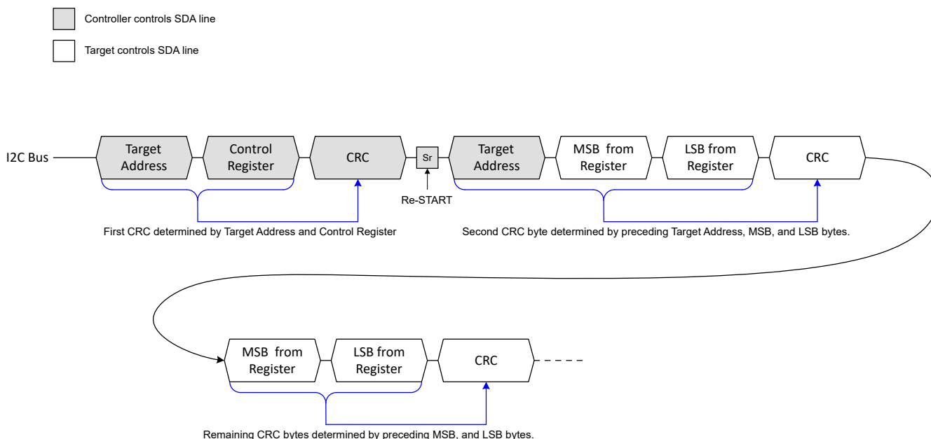
图 8-17. CRC Enabled Read
