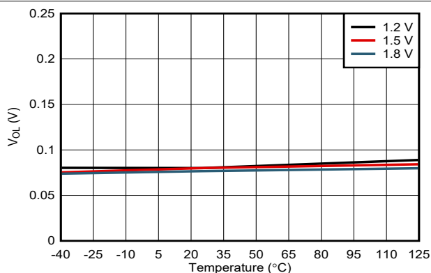
图 7-11. V_{OL} vs. Temperature
