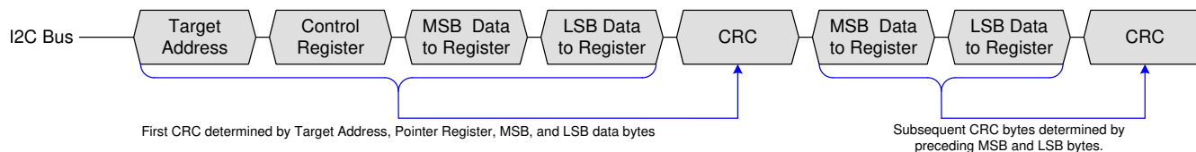
图 8-13. CRC Enabled Write
