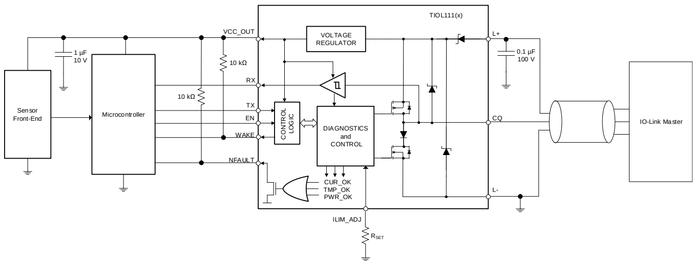
典型应用图
