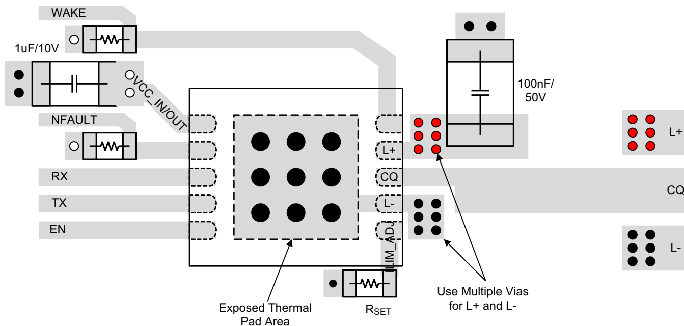
图 31. Layout Example
