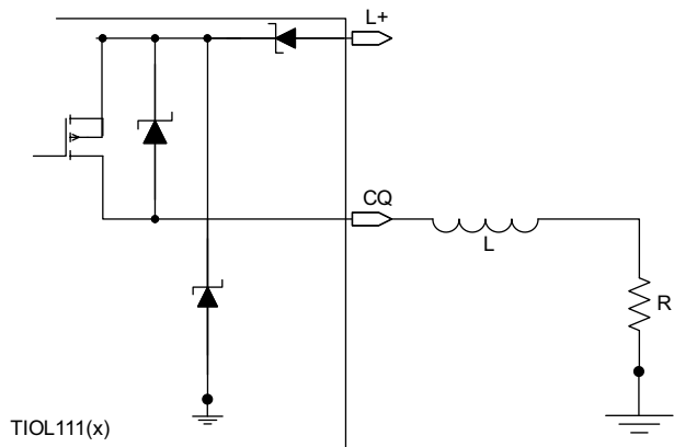
图 18. P-Switch Mode
