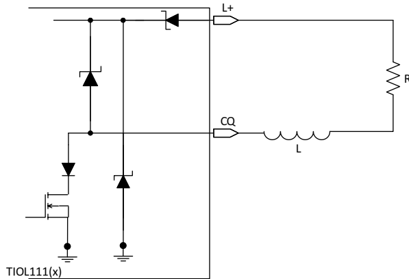
图 19. N-Switch Mode
