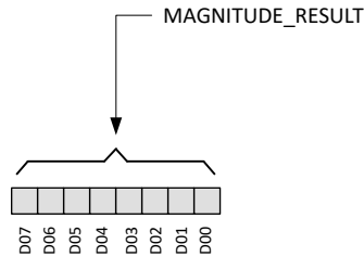
图 7-18. Magnitude Result Data Definition
