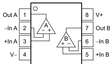
引脚功能 : OPA2348-Q1
