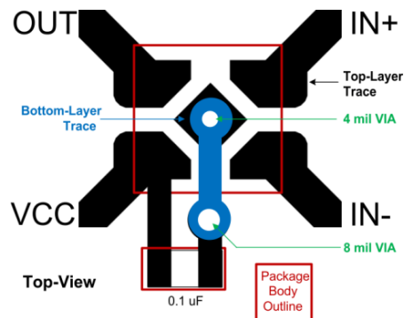
图 48. Layout Example
