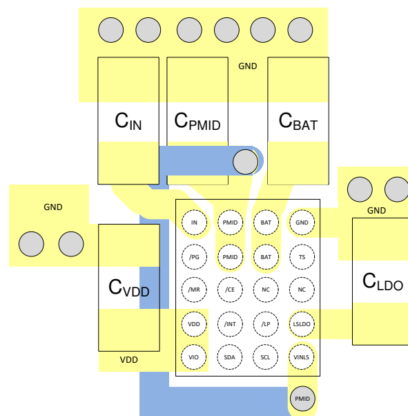
图 81. Layout Example
