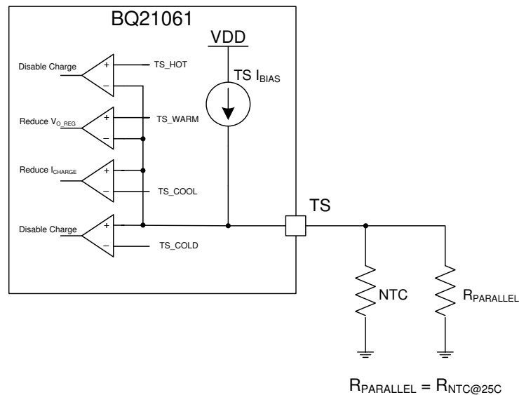
图 23. TS Bias Functional Diagram
