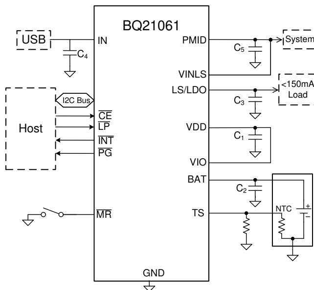
简化原理图
