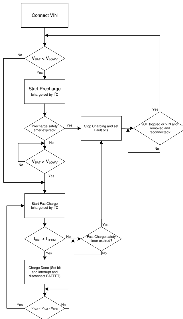
图 16. BQ21061 Charger Flow Diagram
