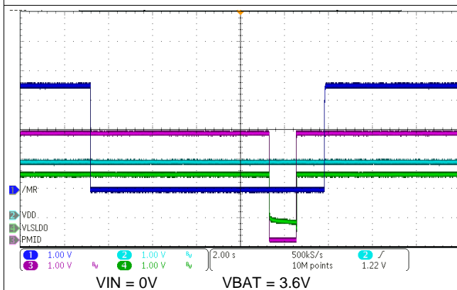
图 66. HW Reset on \overline{MR} Long Button Press
