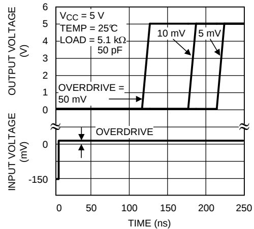
图 14. 传播延迟与过驱电压间的关系
