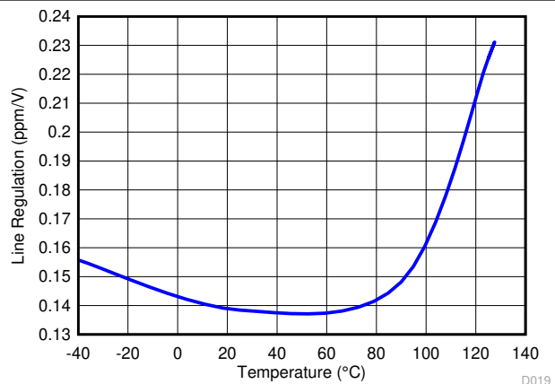
图 7-6. Line Regulation
