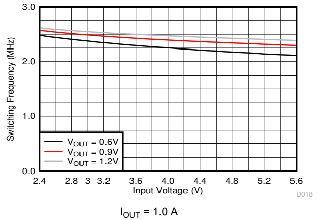
图 9-9. Switching Frequency
