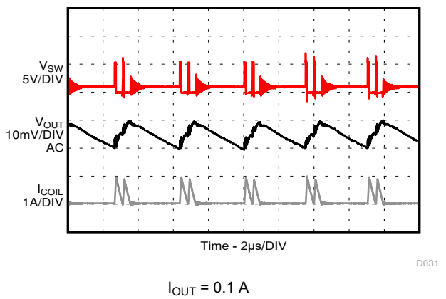
图 9-13. PSM Operation
