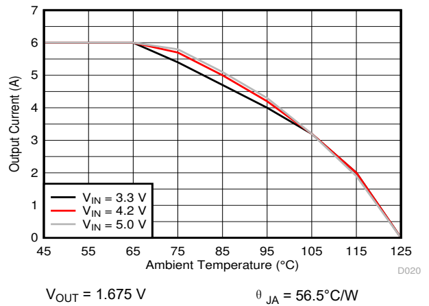
图 9-11. Thermal Derating
