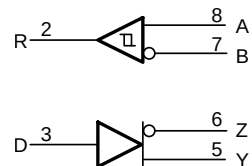
THVD1452 简化原理图
