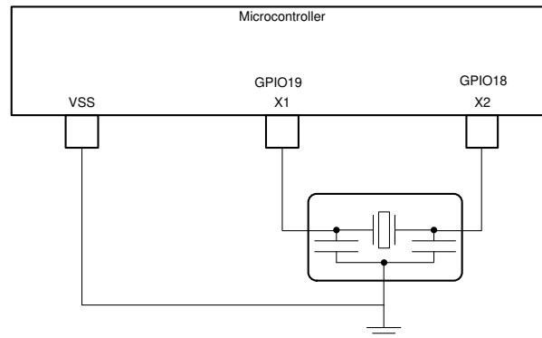
图 7-14. External Resonator
