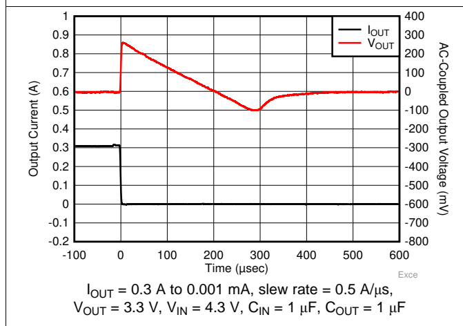
图 29. Load Transient
