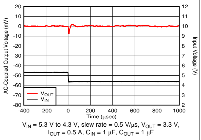
图 30. Line Transient
