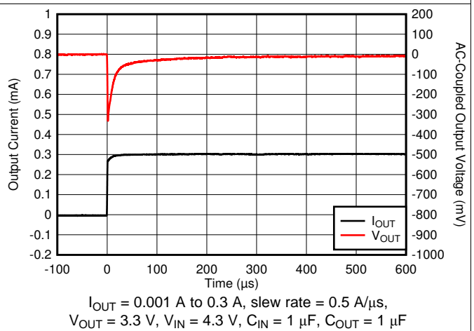
图 28. Load Transient
