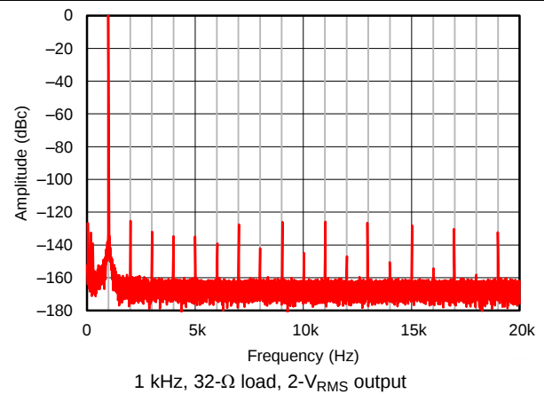
图 45. Output Spectrum
