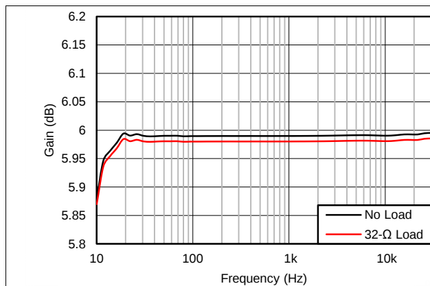
图 42. Amplifier Transfer Function
