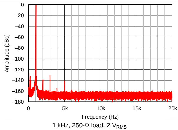
图 46. Output Spectrum
