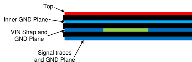
图 10-2. Example Layout for VQFN Package
