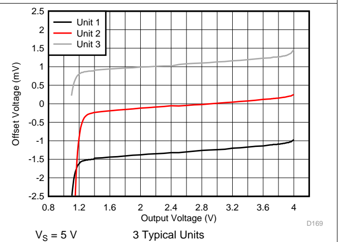
图 36. Offset Voltage vs Output Swing
