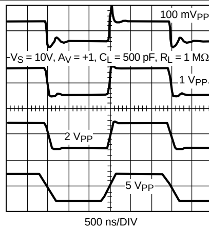
图 38. 各种幅度的阶跃响应
