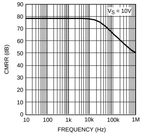
图 34. CMRR 与频率间的关系
