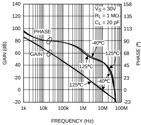
图 31. 不同温度下的开环频率响应
