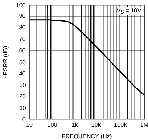
图 35. +PSRR 与频率间的关系
