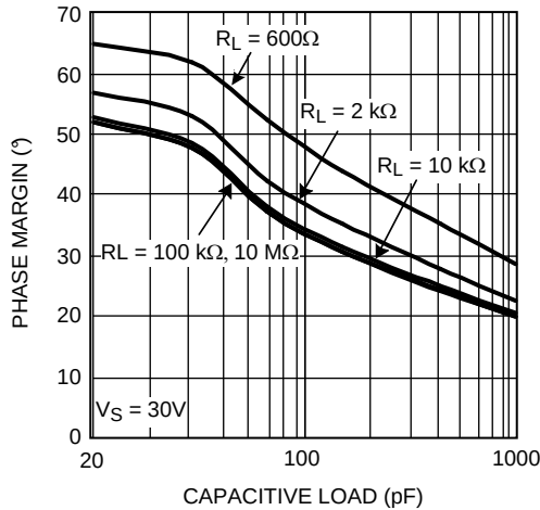
图 33. 相位裕度与容性负载间的关系
