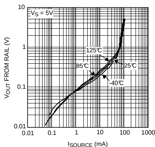
图 20. 输出摆幅与拉电流间的关系
