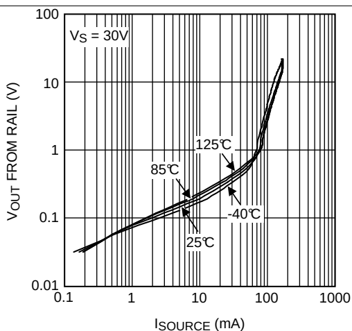
图 21. 输出摆幅与拉电流间的关系
