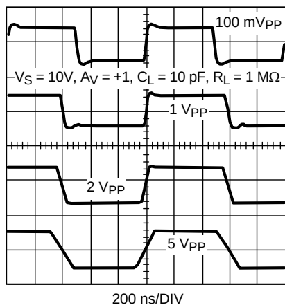
图 37. 各种幅度的阶跃响应
