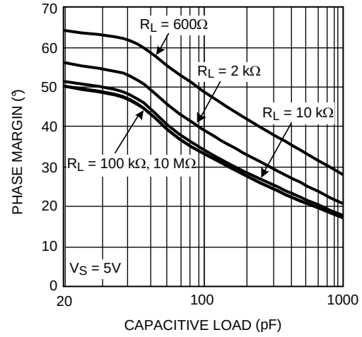
图 32. 相位裕度与容性负载间的关系
