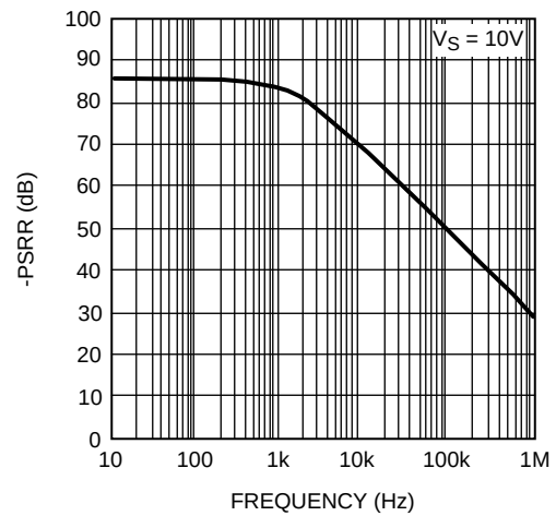
图 36. -PSRR 与频率间的关系
