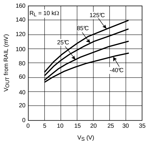
图 23. 正输出摆幅与电源电压间的关系
