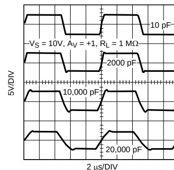
各种容性负载的大信号阶跃响应
