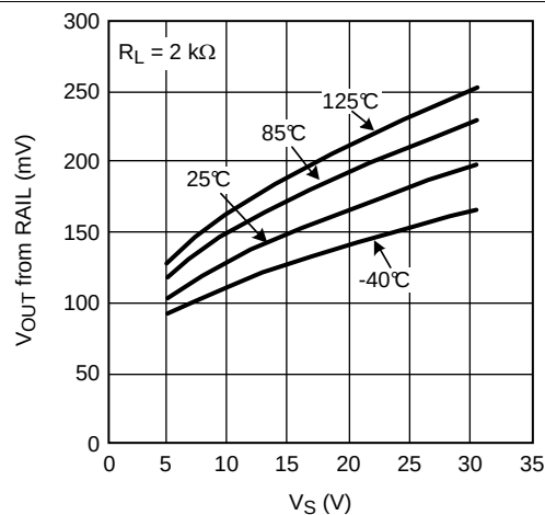
图 22. 正输出摆幅与电源电压间的关系
