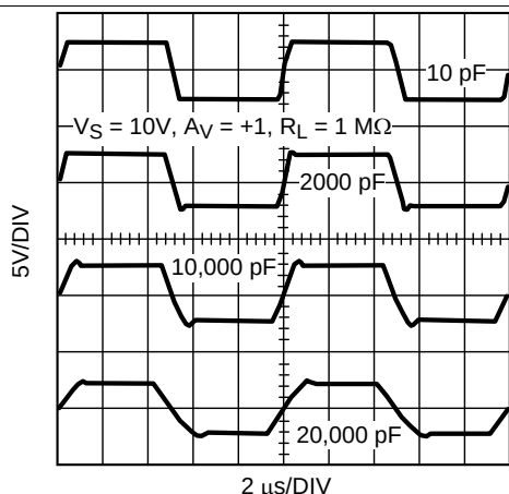
图 39. 各种容性负载的大信号阶跃响应
