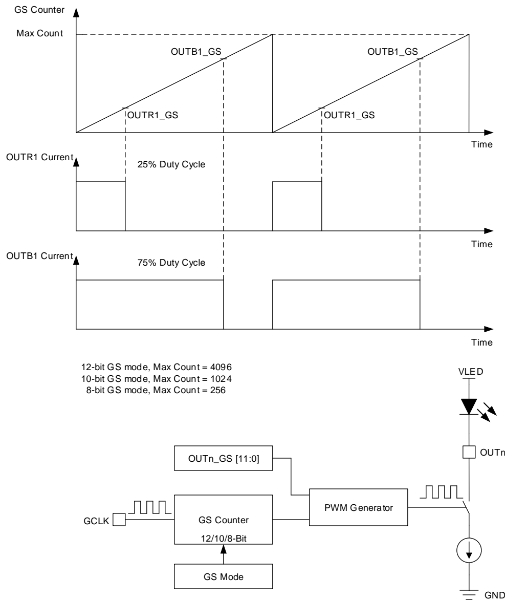
图 22. PWM Generator
