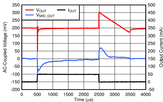
图 6-27. Load Transient
