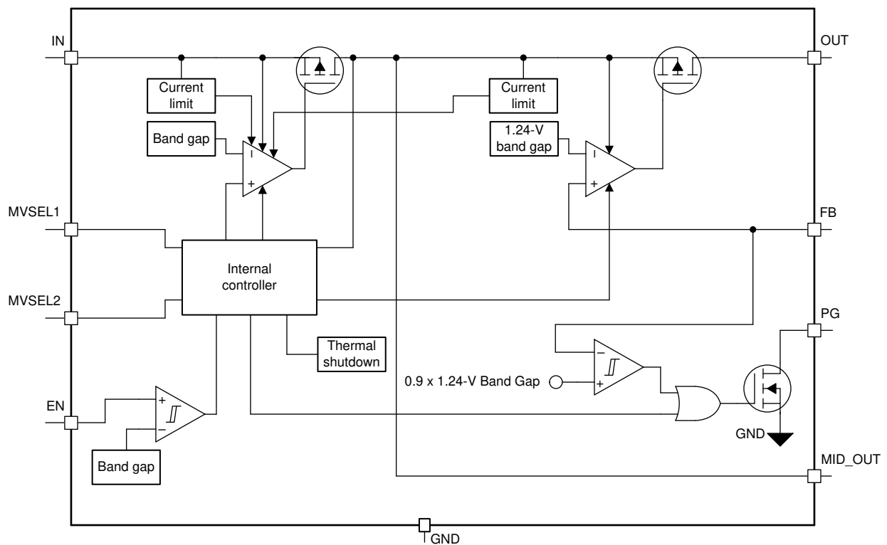
图 7-1. Adjustable Version
