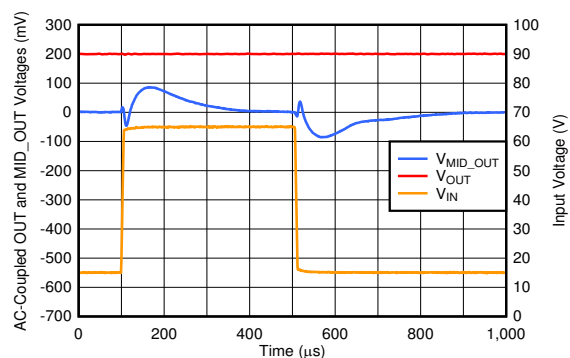
V_{MID\_OUT} = 12V 、 V_{OUT} = 3.3V 、 I_{OUT} = 50mA 时的线路瞬态
