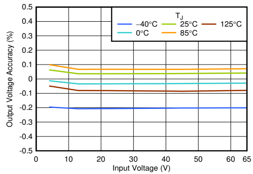
图 6-2. V_{OUT} Accuracy vs V_{IN}
