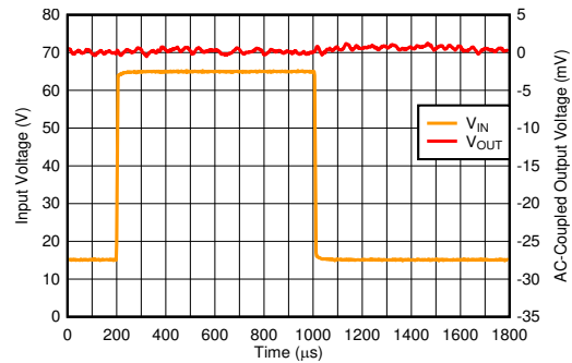
图 6-20. Line Transient
