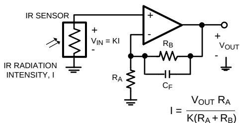
图 60. 红外辐射传感器
