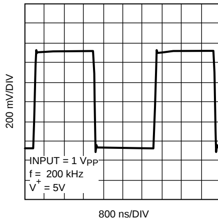
图 39. 大信号瞬态响应
