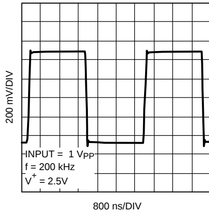
图 37. 大信号瞬态响应
