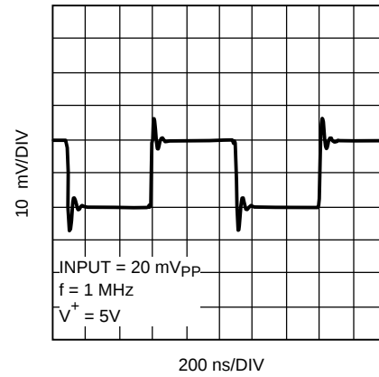
图 38. 小信号瞬态响应
