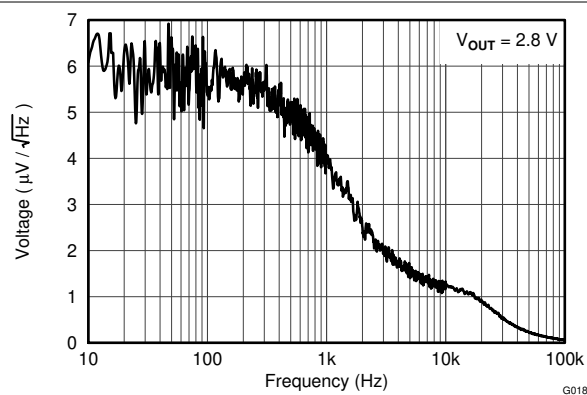
图 6-19. Noise
