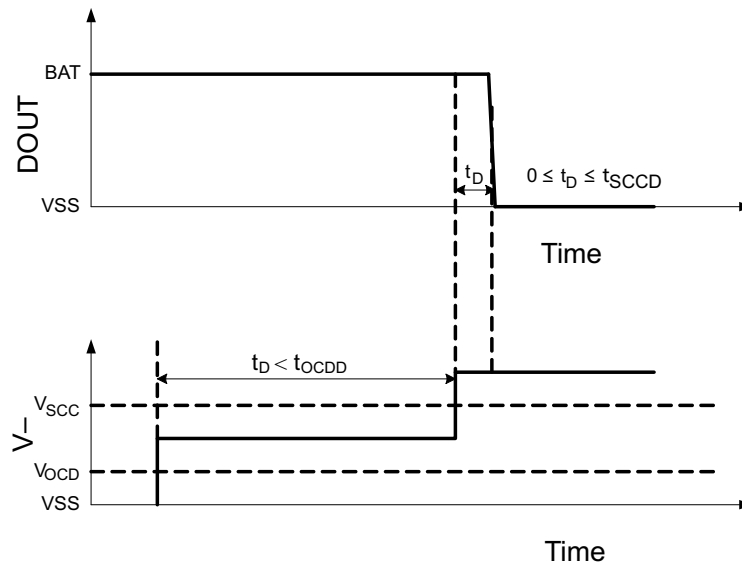
图 9-1. Delay Circuit
