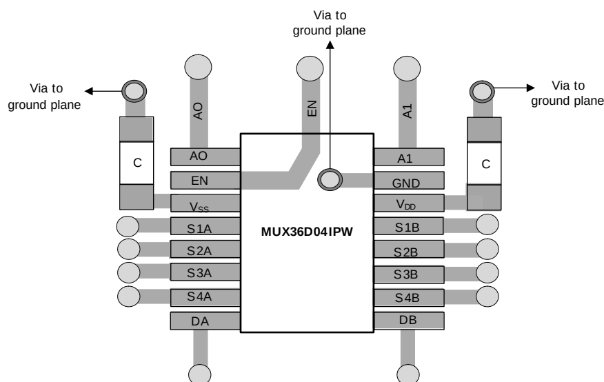
图 47. MUX36D04IPW Layout Example
