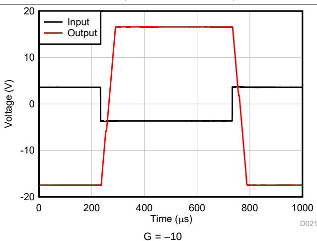
图 28. Overload Recovery
