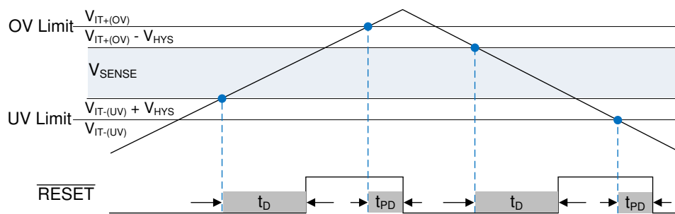
图 23. \overline{\text{RESET}} output
