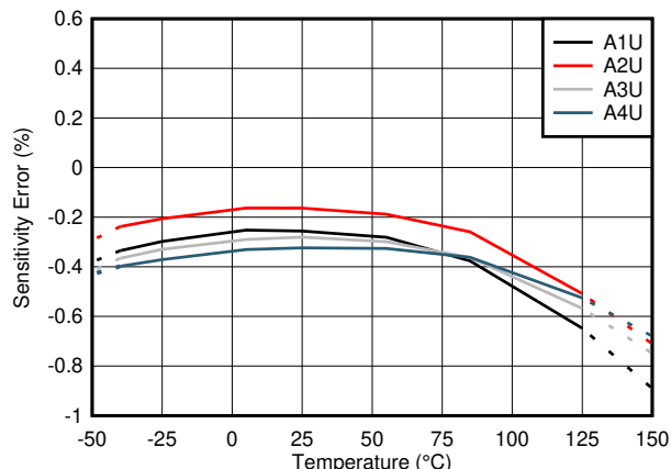
图 7-2. TMCS1101AxU-Q1 Sensitivity Error vs Temperature
