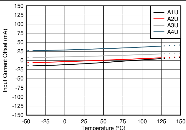
图 7-4. TMCS1101AxU-Q1 Input Offset Current vs Temperature
