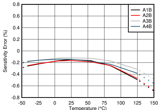
图 7-1. TMCS1101AxB-Q1 Sensitivity Error vs Temperature
