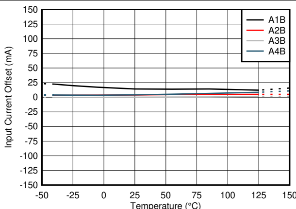
图 7-3. TMCS1101AxB-Q1 Input Offset Current vs Temperature
