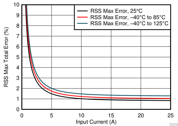
图 10-1. RSS Error vs. Input Current
