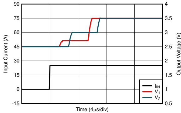
图 7-23. Voltage Output Step, Rising
