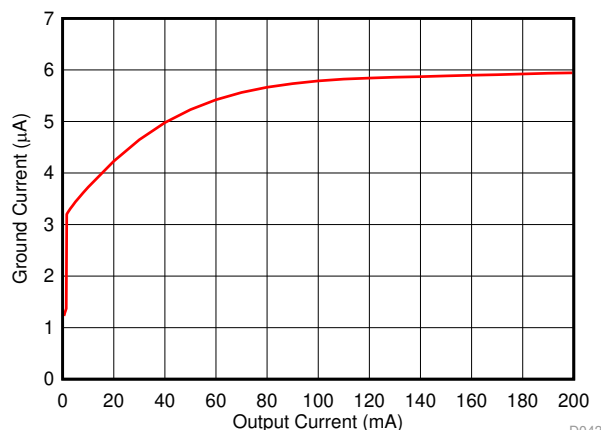
接地电流与输出电流间的关系
