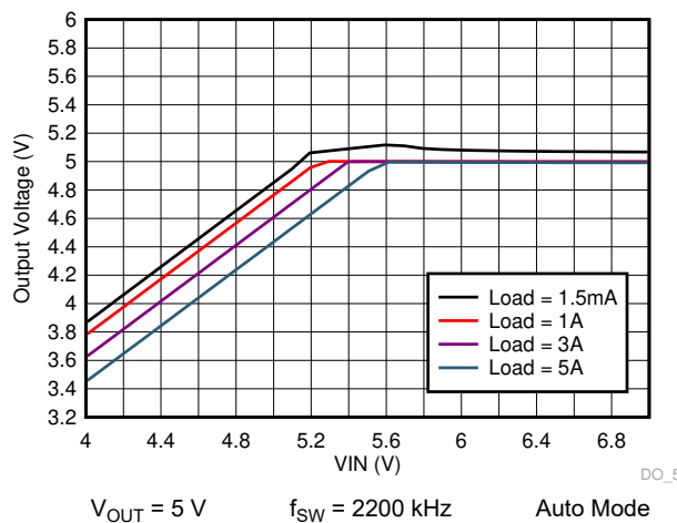
图 9-37. LM73605-Q1 Dropout Curve
