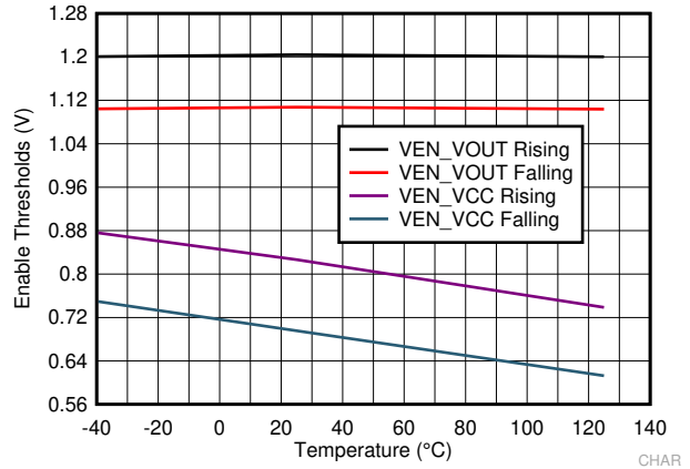
图 7-8. Enable Thresholds
