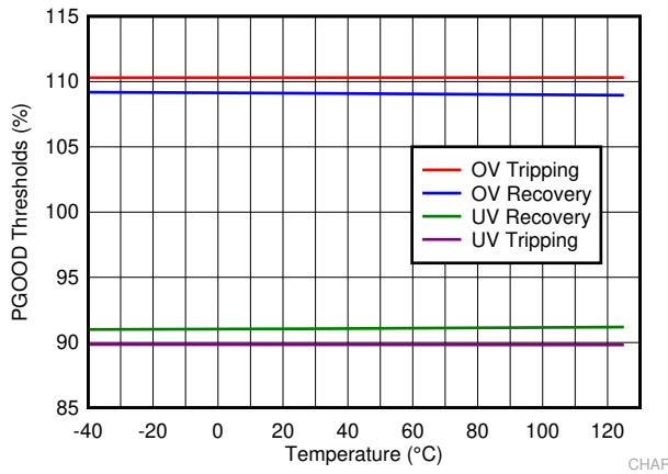
图 7-9. PGOOD Thresholds
