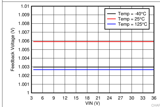
图 7-3. Feedback Voltage
