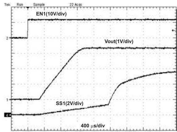
Figure 10. VO1=3.3V, SoftStart
