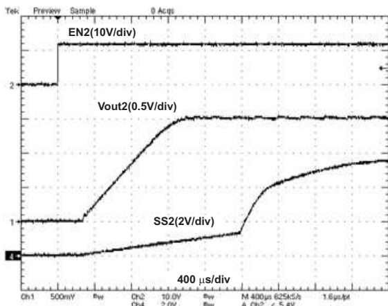
Figure 11. VO2=1.5V, SoftStart
