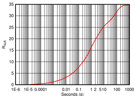
图 3. Transient Thermal Impedance 1 Channel Enabled
