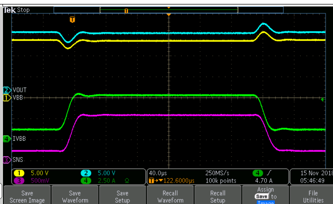
图 28. I_{SNS} Settling time ( t_{SNSION1} ) on Load Step
