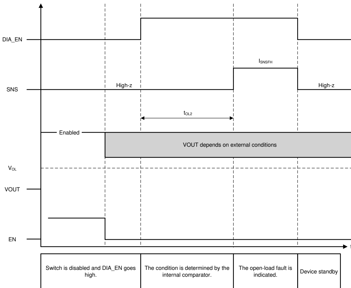
图 42. Open Load
