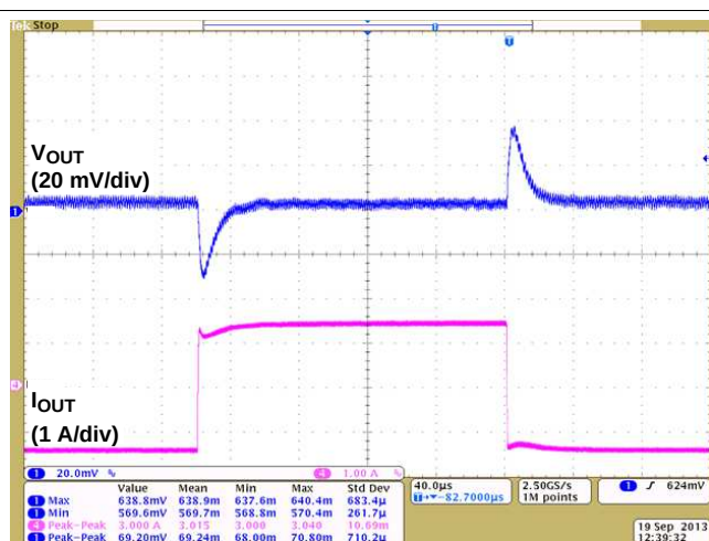
图 32. Load Transient
