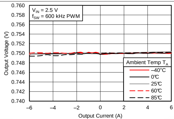
图 8. Load Regulation
