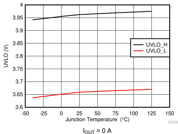
图 6-12. UVLO Threshold
