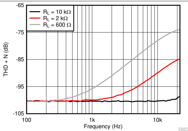
D023 V_{OUT} = 0.5\text{ V}_{RMS} G = +1 V_{CM} = 2.5\text{ V} BW = 80\text{ kHz}
