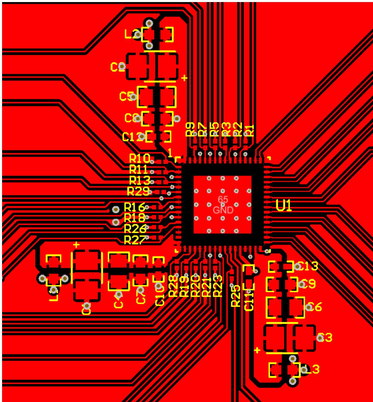
图 19. Layout Example
